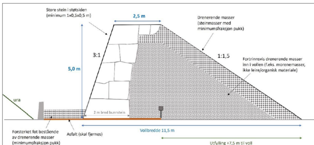
Figur 28: Prinsippskisse av anbefalt utforming av fangvoll. Dette snittet viser utformingen i delstrekning C, der vollen blir 5 – 5,5 meter høy og vollkrona 2,5 meter bred..
